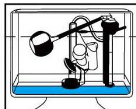
Chasse d'eau d'une toilette sans l'économiseur d'eau EcoWC, le réservoir se vide complètement.
